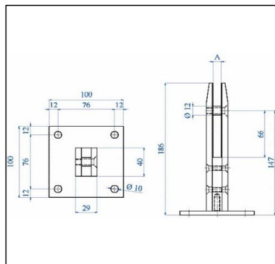
Bodenglashalter Rechteckig für Glasstärke 12 - 17.52mm
